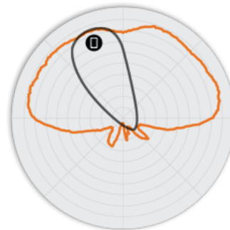
Figure 4. Diagrammes d'antennes Élévation T350c/d 2,4 GHz
