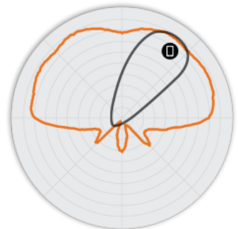
Figure 5. Diagrammes d'antennes Élévation T350c/d 5 GHz
