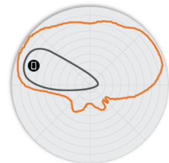
Figure 5. Diagrammes d'antennes Élévation T750 5 GHz
