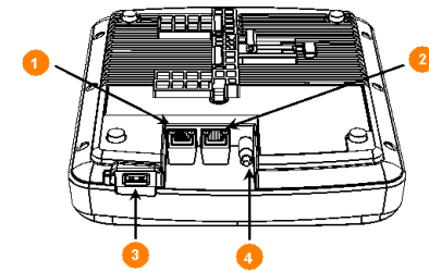
FIGURE 1 Ports du point d'accès R650
