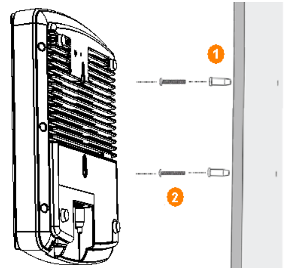
FIGURE 5 Montage sur surface plate
