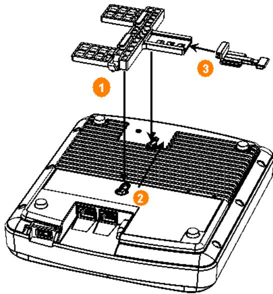
FIGURE 3 Fixation du support de fixation pour barre en T au point d'accès
