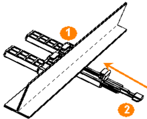
FIGURE 4 Fixation du support de fixation pour barre en T à la barre en T
