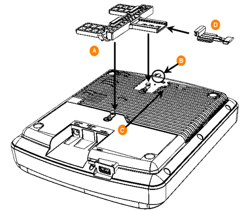
FIGURE 3 Fixation du support de fixation pour barre en T au point d'accès
