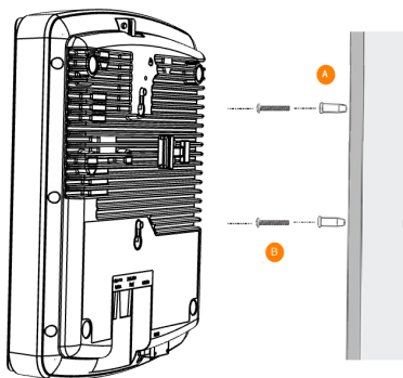
FIGURE 5 Montage sur surface plate
