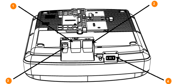
FIGURE 1 Éléments du panneau inférieur du R750
