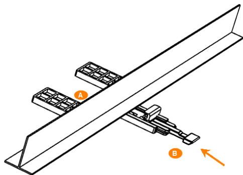
FIGURE 4 Fixation du support de fixation pour barre en T à la barre en T
